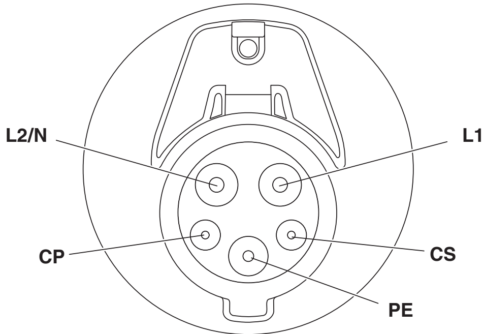
Esquema de polos de entradas de carga para vehículos
