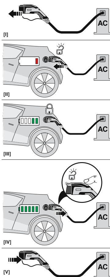
Dibujo funcional
