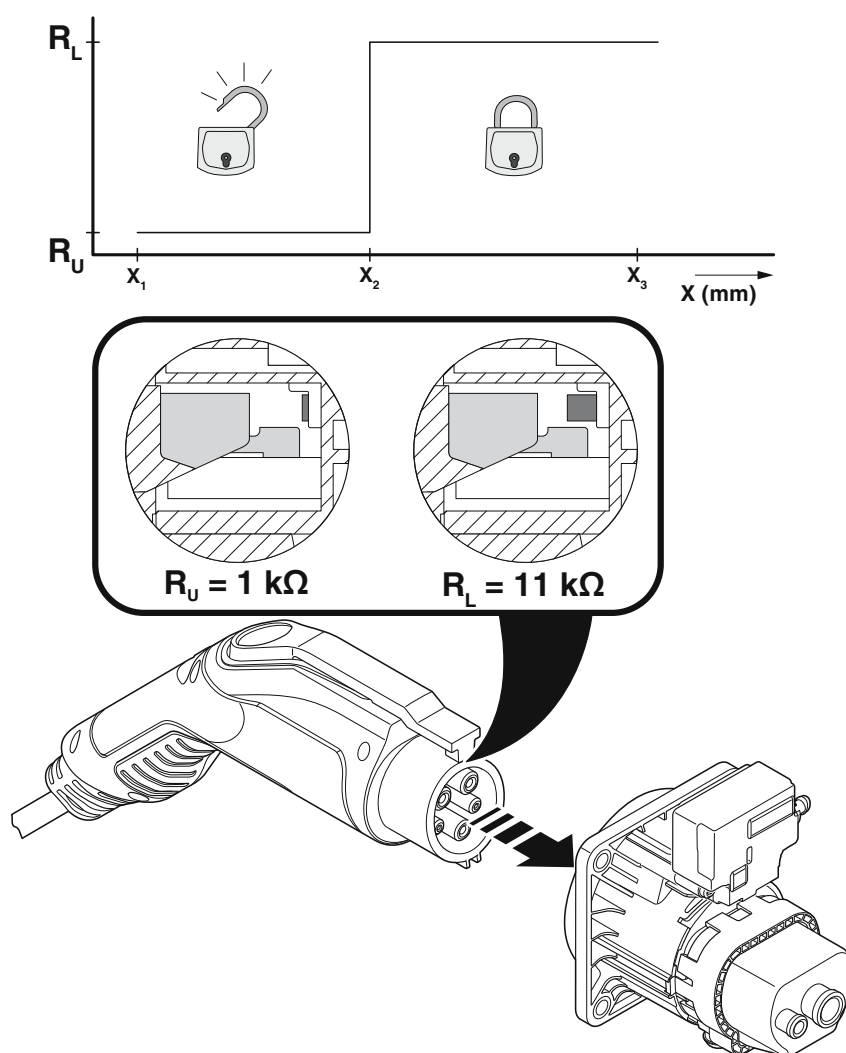
Plano esquemático
