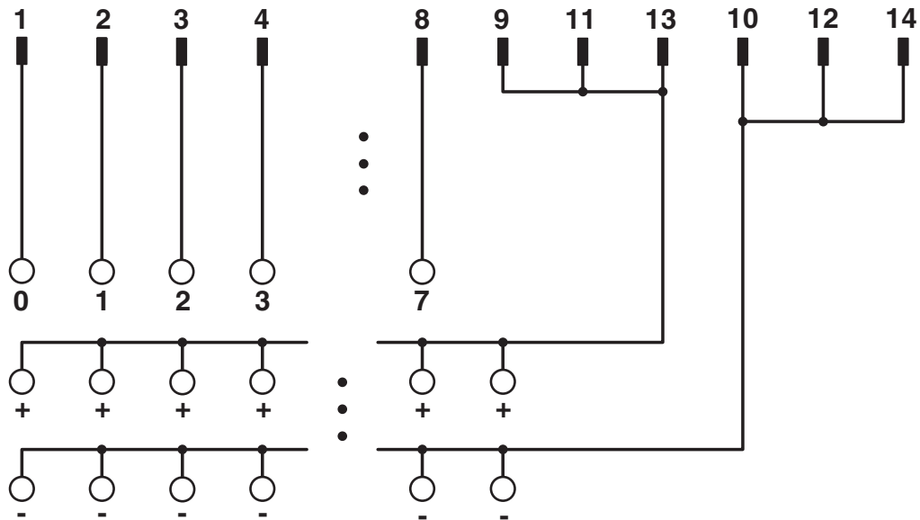
Diagrama eléctrico
