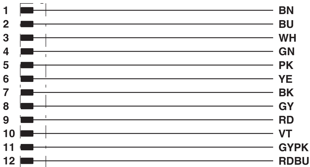
Kontaktbelegung der M12-Stecker
