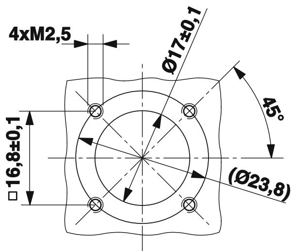
Maßzeichnung
