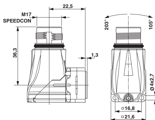
Maßzeichnung
