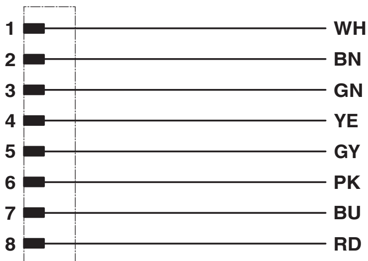
Ocupación de contactos del conector macho M12
