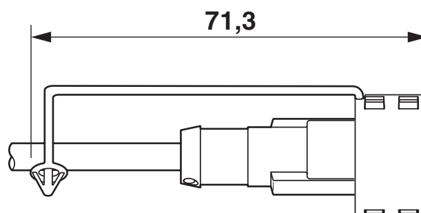
Maßzeichnung
