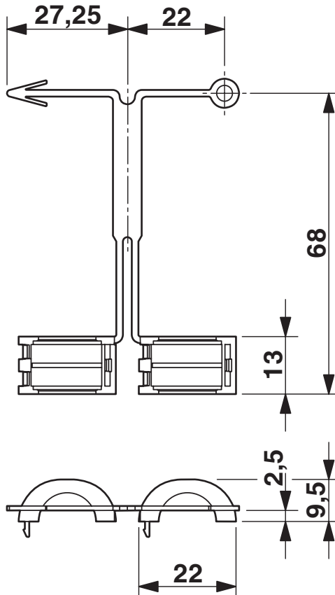
Maßzeichnung
