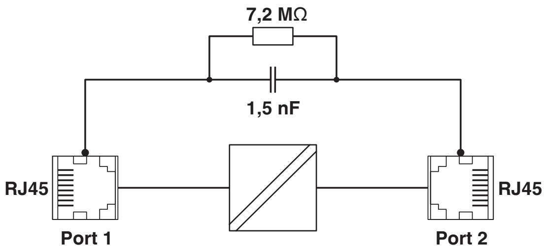
Schéma fonctionnel
