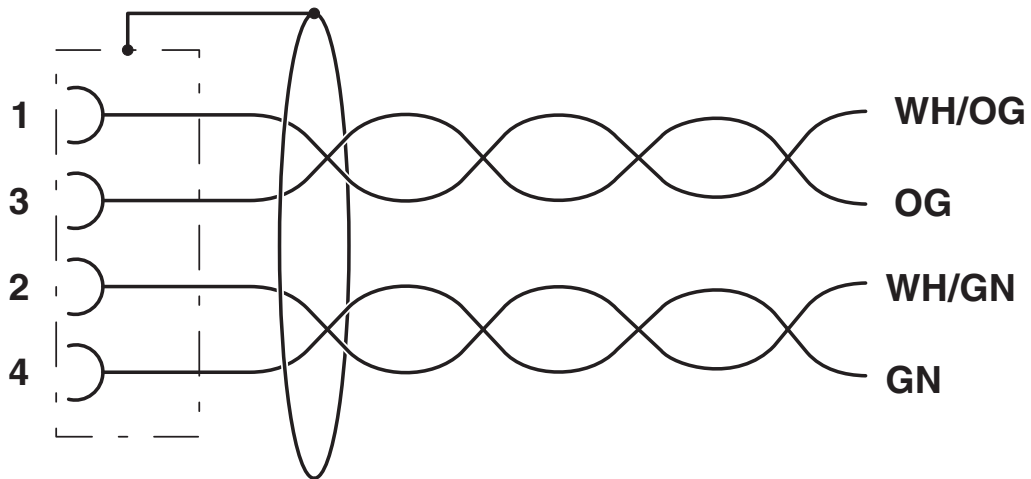
Diagrama eléctrico
