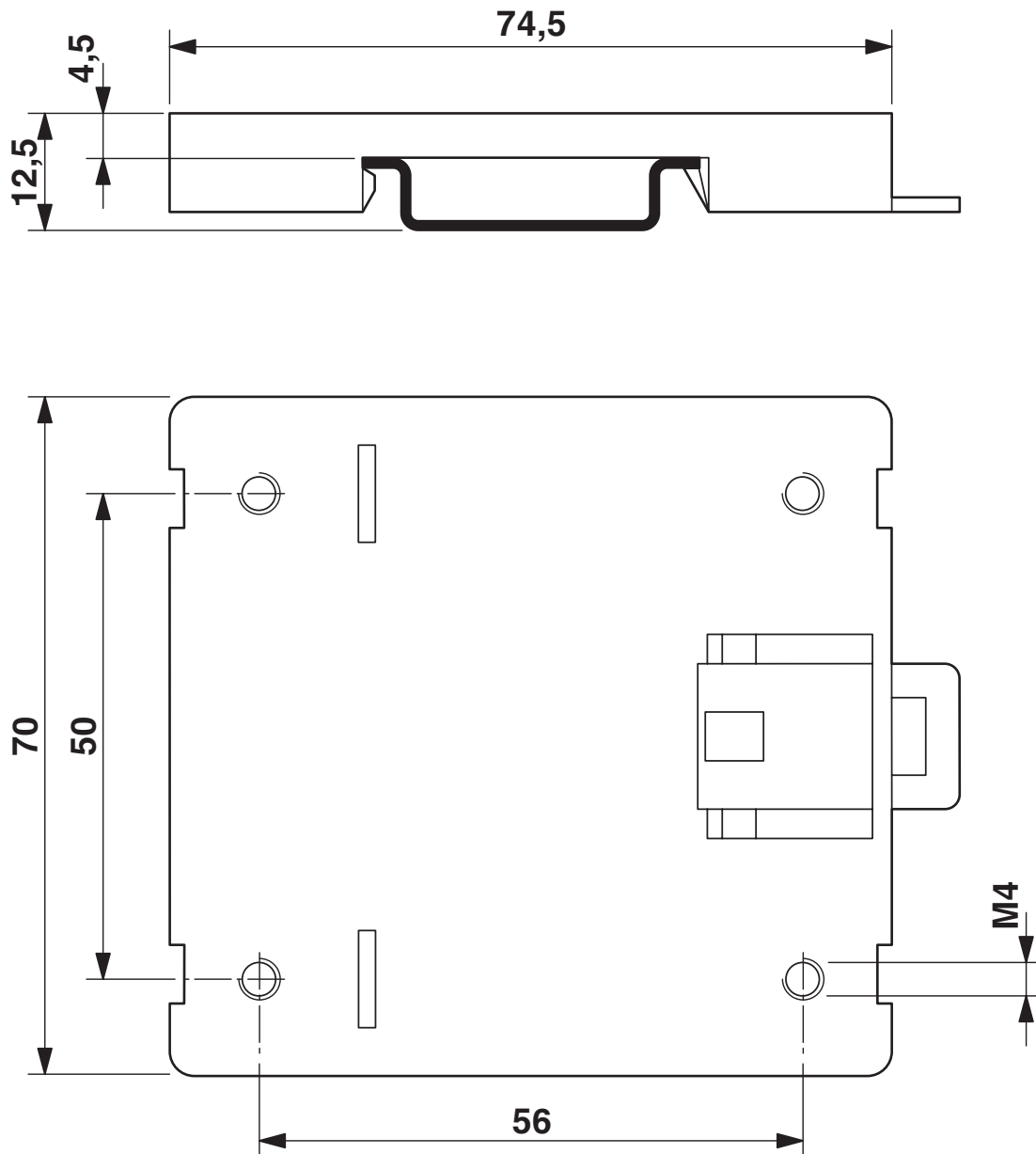
Maßzeichnung
