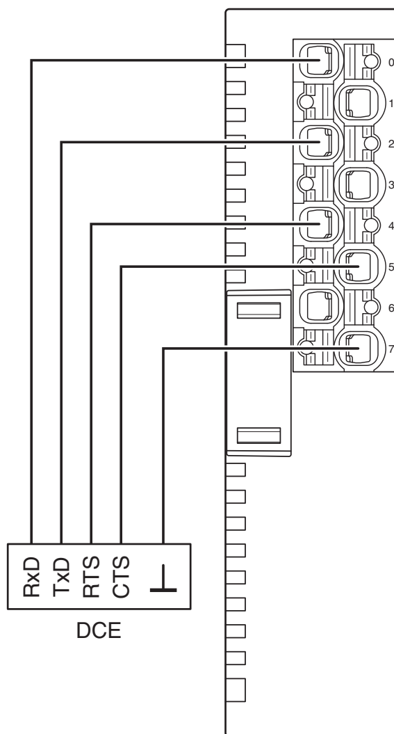
Dessin de la connexion
