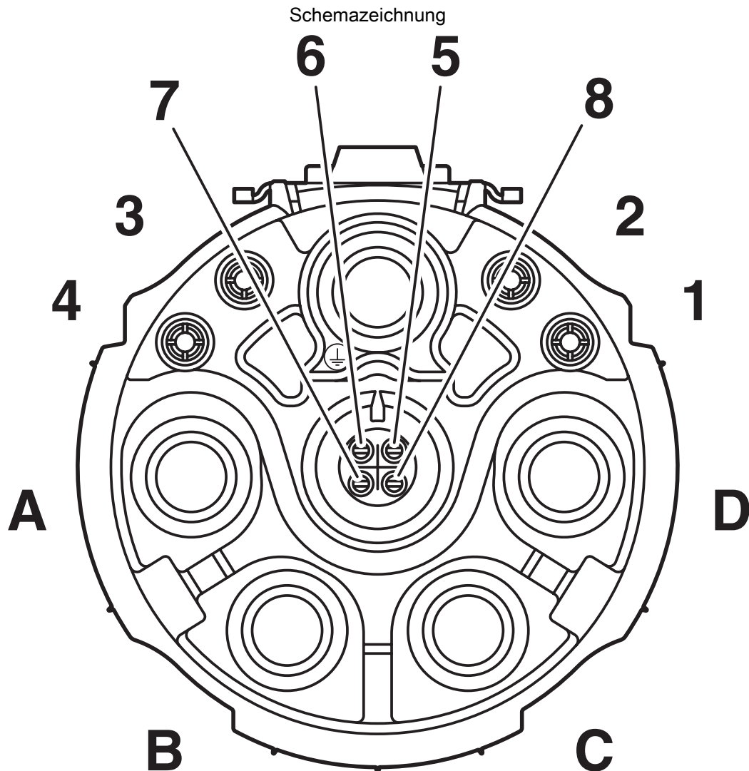
Polbild Buchse CAT5, Kodierung 1
