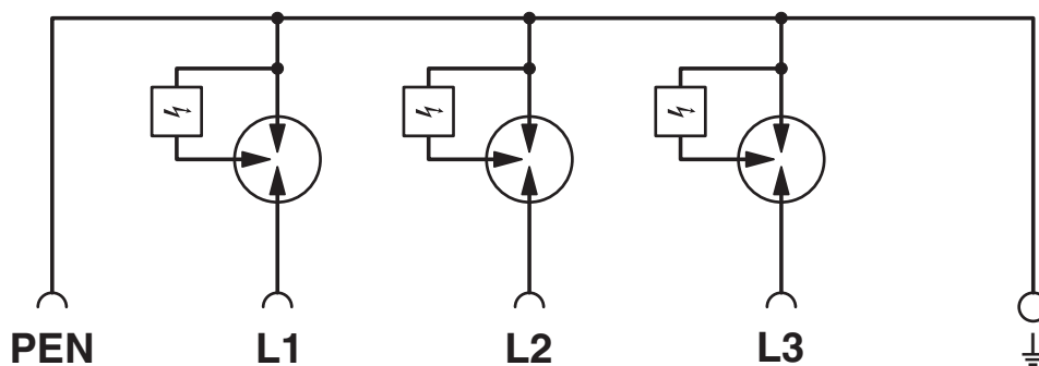
Schaltplan
