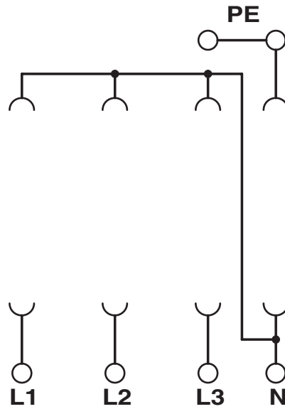
Schaltplan
