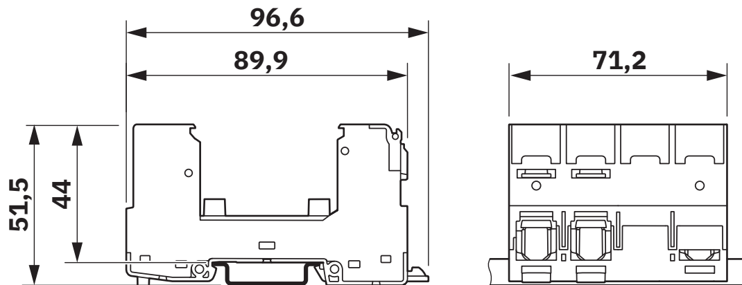
Maßzeichnung
