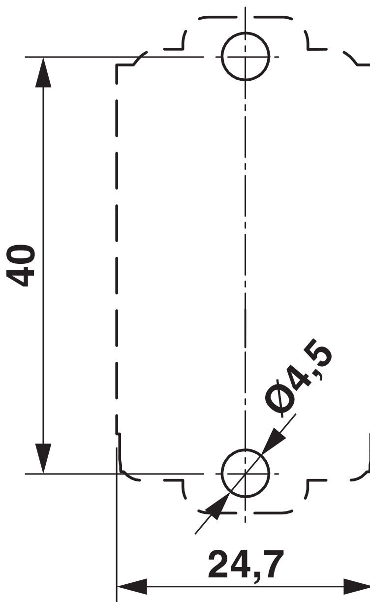
Gabarit perçage / géom. pastille soudage
