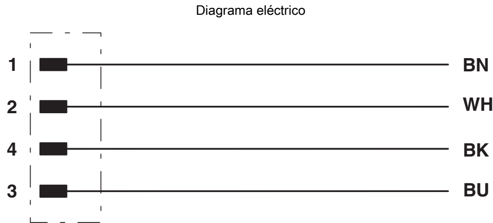
Ocupación de contactos del conector macho M12
