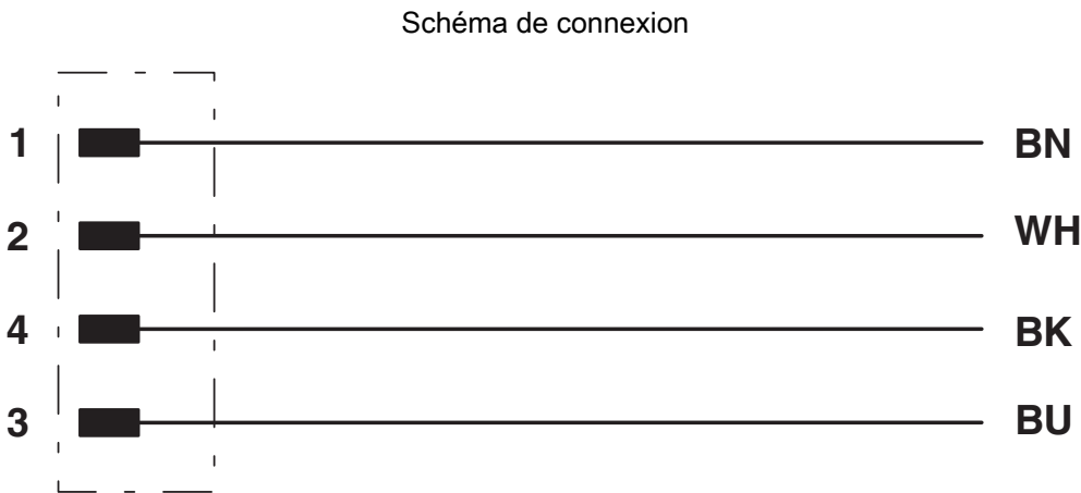
Affectation des contacts du connecteur mâle M12
