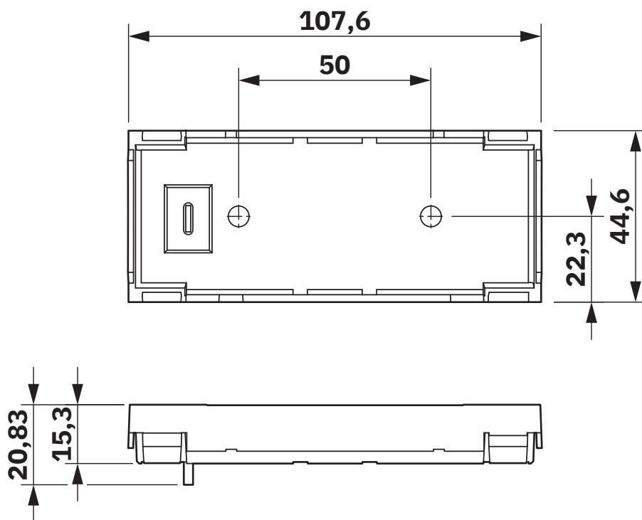
Maßzeichnung
