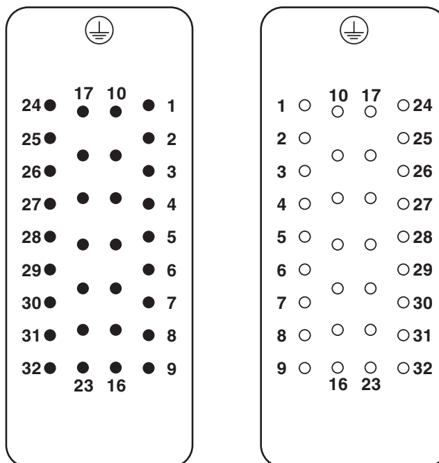
Dessin schématique
