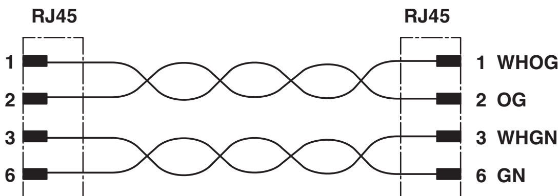
Ocupación de contactos de los conectores macho RJ45
