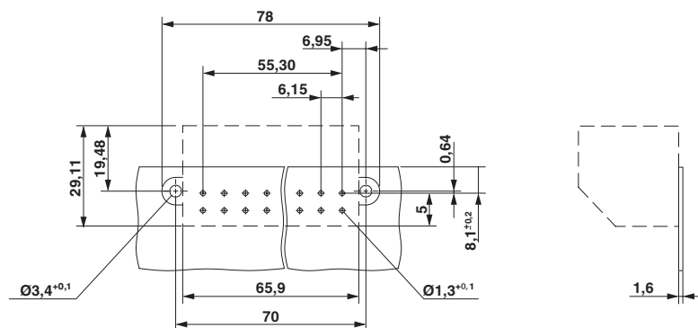
Dessin coté
