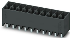
Abbildung zeigt eine 10-polige Variante mit 20 Kontakten
