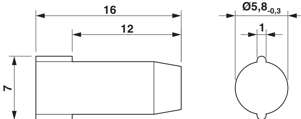
Dessin coté
