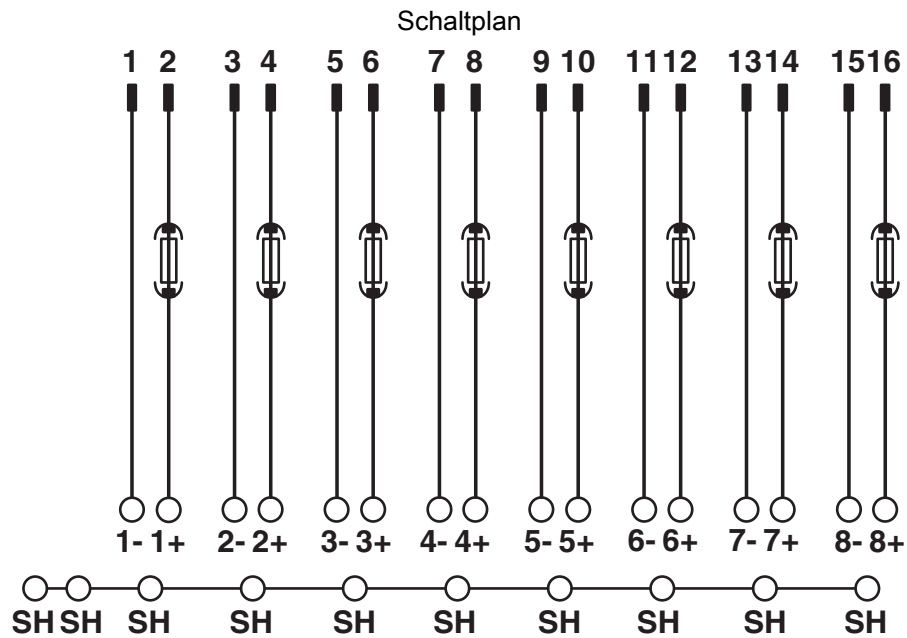
Anschlussbild UM-DELTA V/D/SI/BFI/TP
