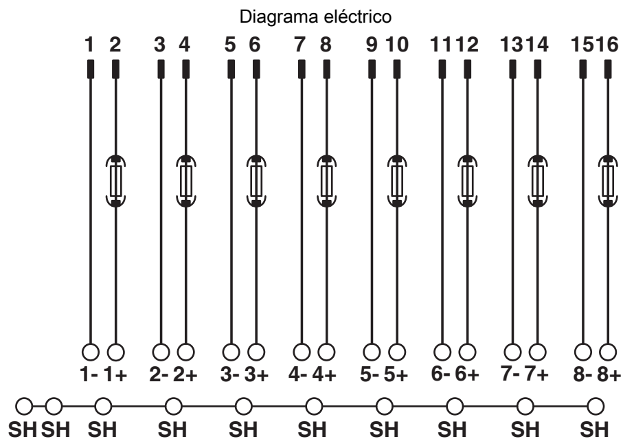
Esquema de conexiones UM-DELTAV/D/SI/BFI/TP
