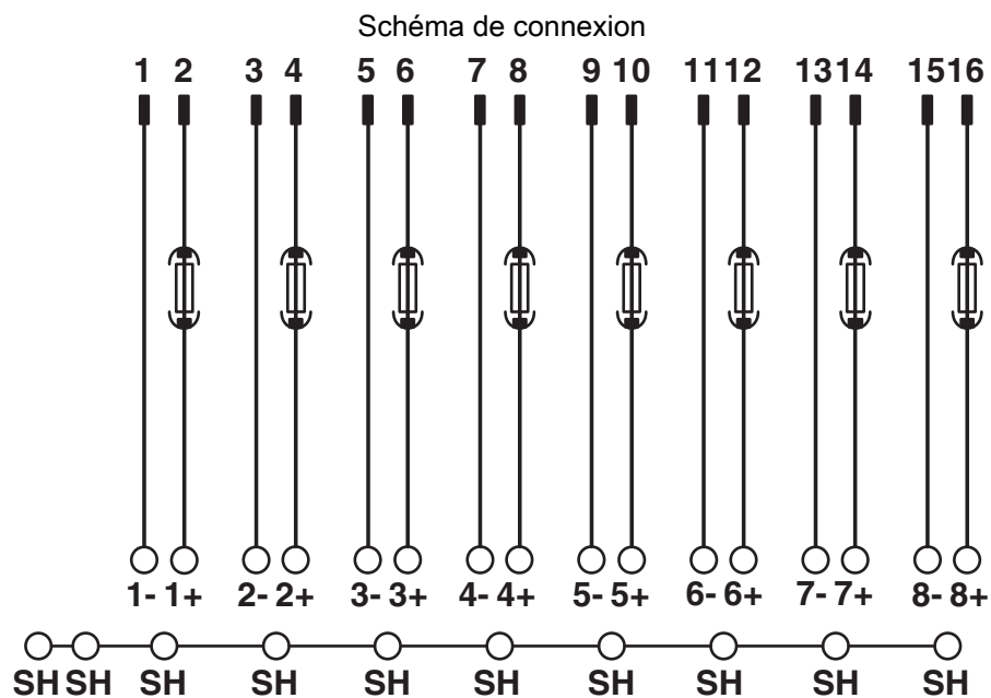
Schéma des connexions UM-DELTAV/D/SI/BFI/TP
