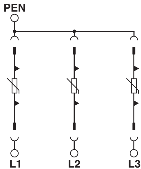
Schaltplan
