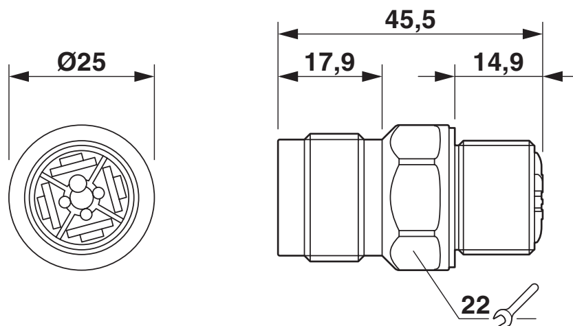
Maßzeichnung
