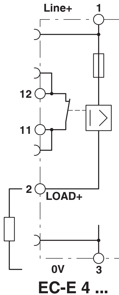
Diagrama eléctrico
