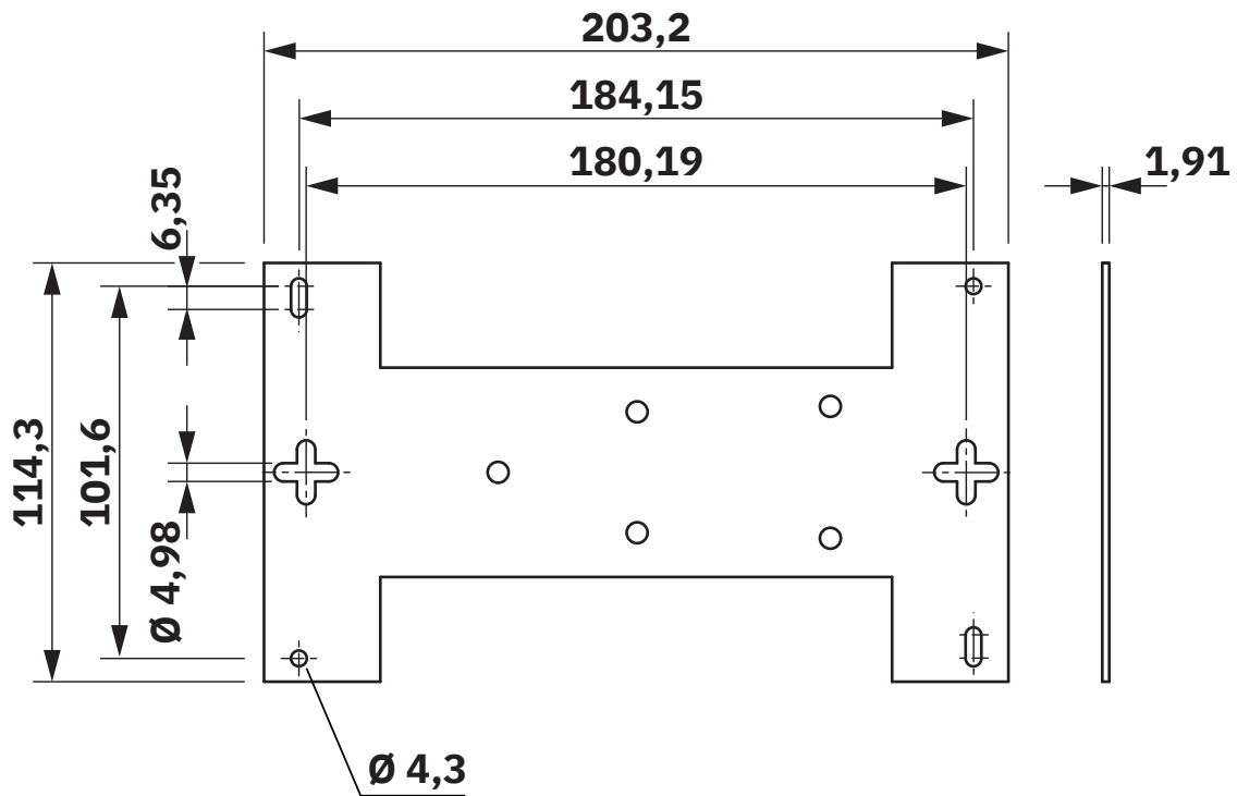
Maßzeichnung
