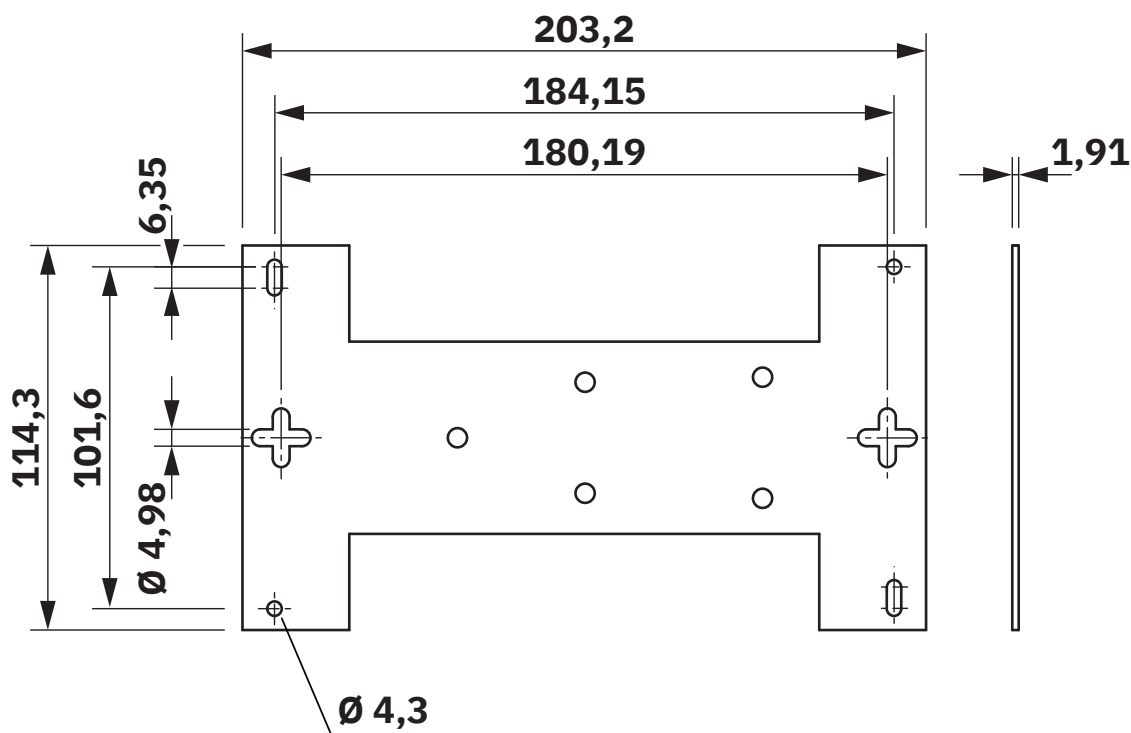
Dessin coté
