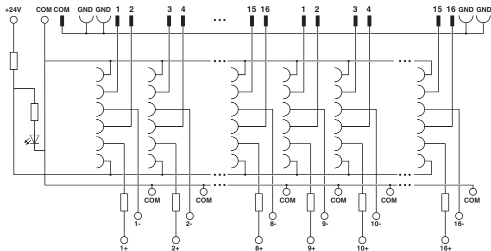
Diagrama eléctrico
