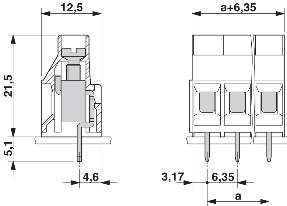
Maßzeichnung
