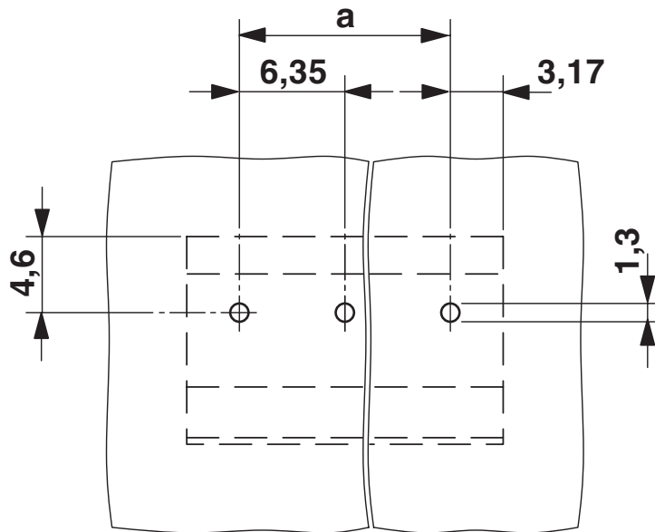
Bohrplan/Lötpadgeometrie
