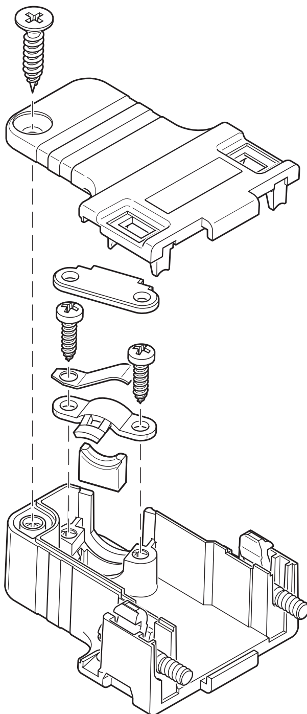
Plano esquemático
