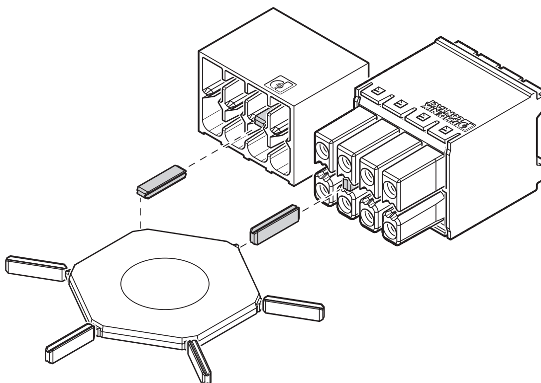
Plano esquemático
