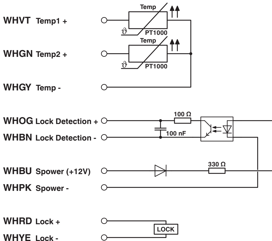
Blockschaltbild GB/T DC
