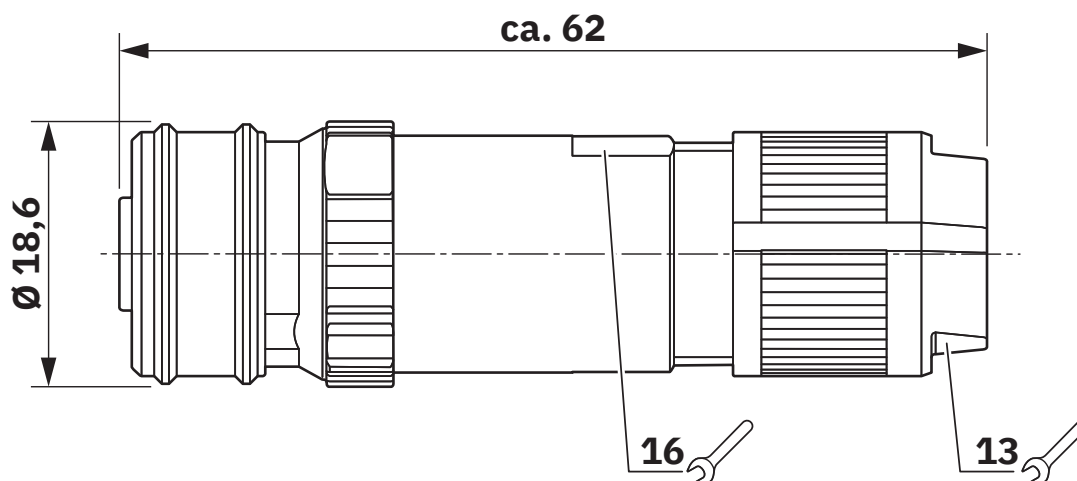
Maßzeichnung
