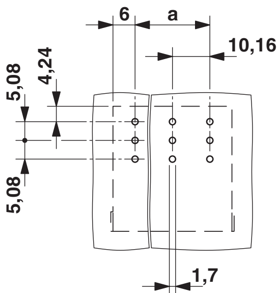
Bohrplan/Lötpadgeometrie
