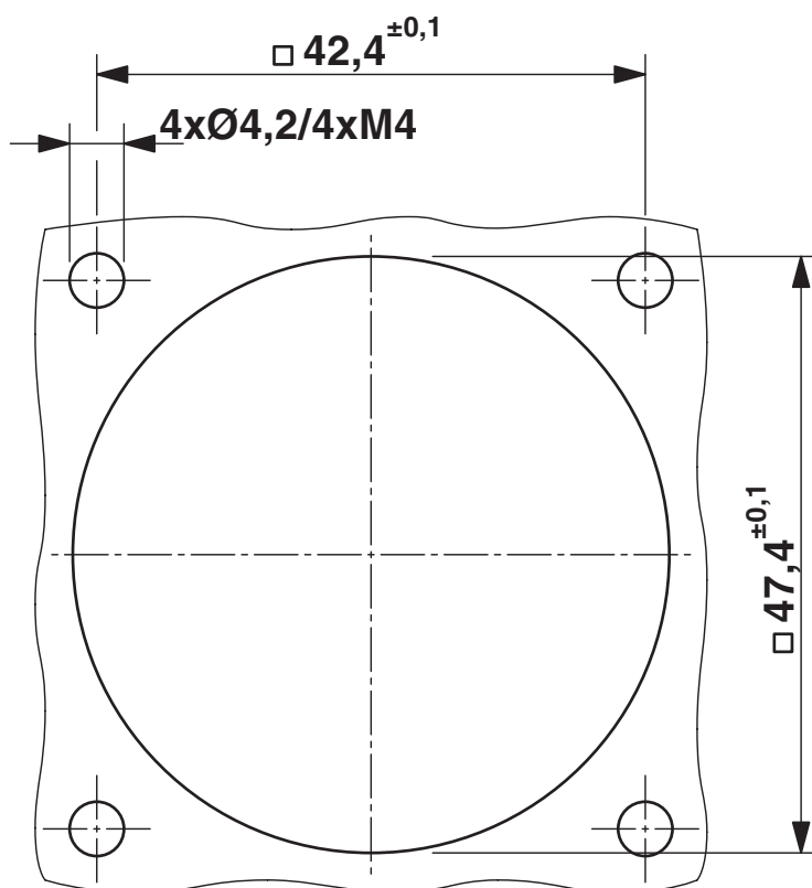
Dessin coté
