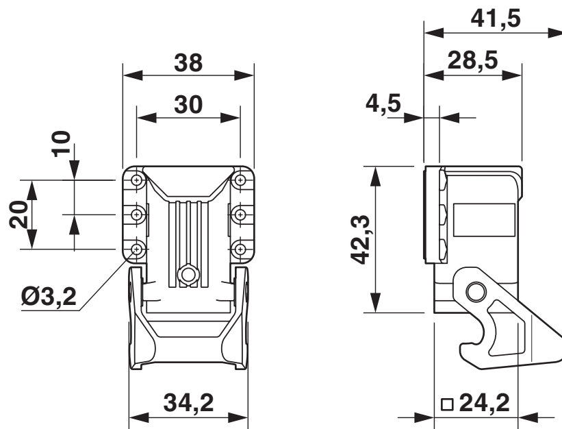
Maßzeichnung
