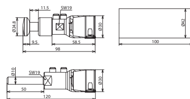
Maßbild HVI P LO ASS KF 27 V2A
