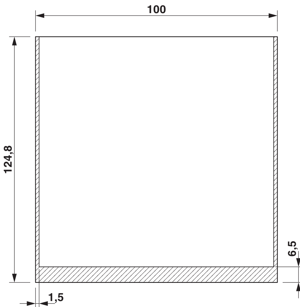
Dessin coté
