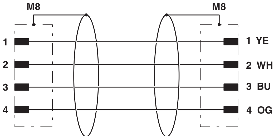
Kontaktbelegung der M8-Stecker
