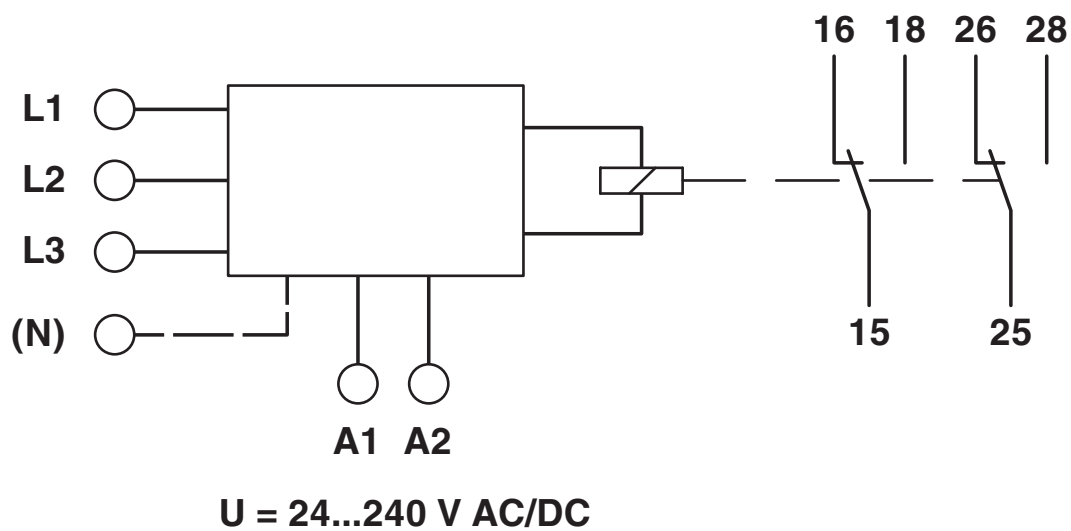
Schéma fonctionnel
