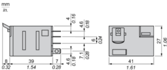
Vista lateral de los pins
