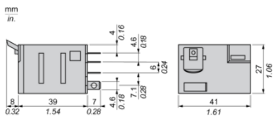
Stecker-Seitenansicht
