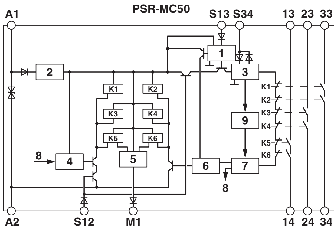
Schéma fonctionnel
