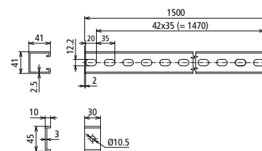
Maßbild MSC MDH V4A L1500 MZ V2A
