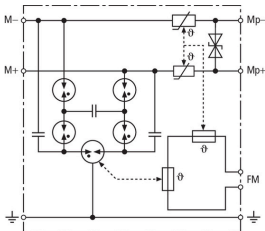
Esquema del BVT KKS APD 36
