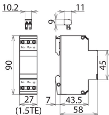
Dimensiones del BVT KKS APD 36
