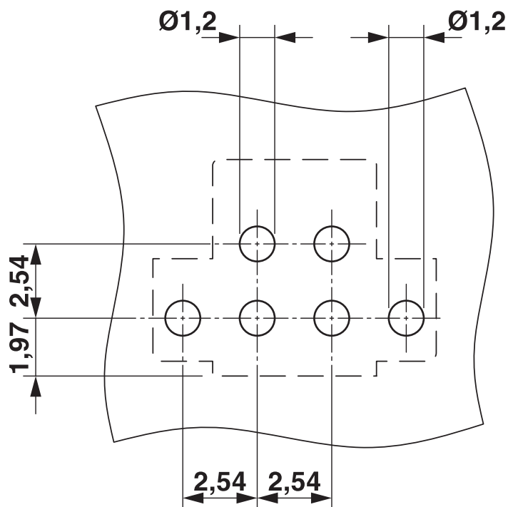
Esquema de taladros/geometría pads soldadura
