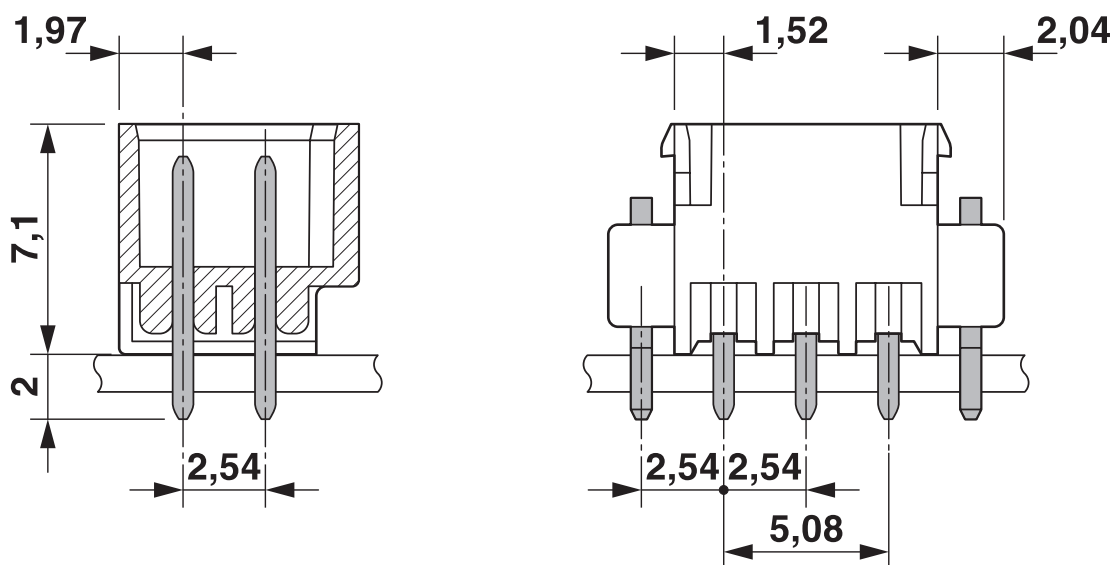
Dessin coté
